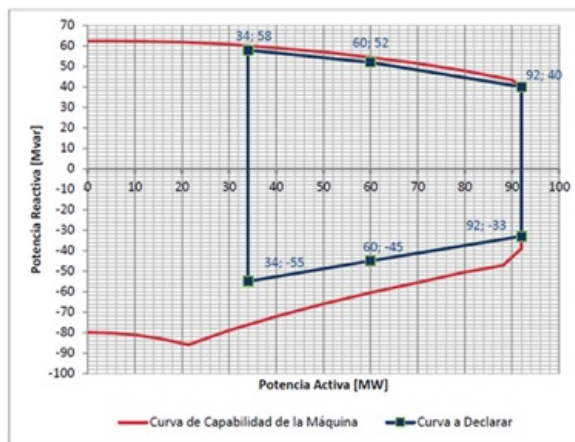
Figura 3. Curva de Carga Unidades de la central Paraiso
