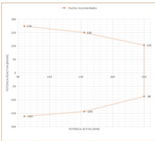
Figura 1: Curva de Carga Unidad 2 Central Guavio
