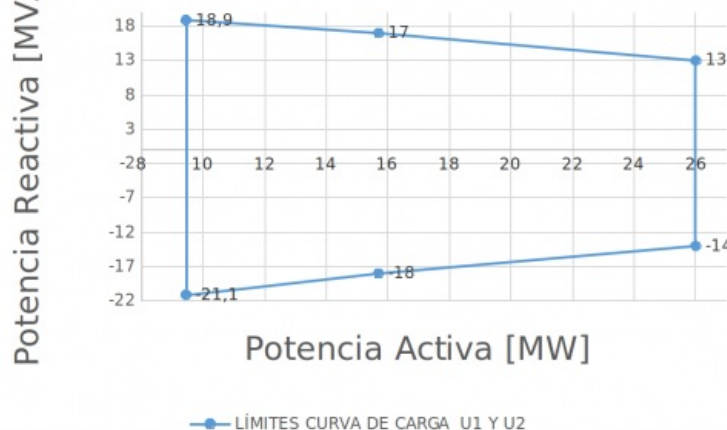
LÍMITES CURVA DE CARGA - UNIDADES 1 Y 2 CENTRAL SAN MIGUEL
